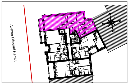
HALL B APPARTEMENT DE 4 PIECES B304 au 3ème étage
