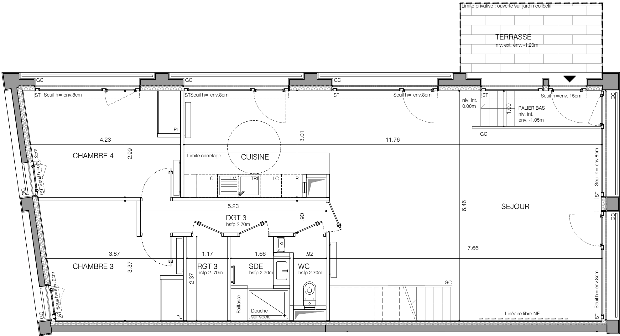
Niveau bas duplex H=env 3.7m
