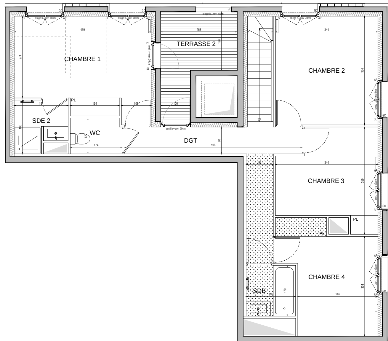
ETAGE HAUT
